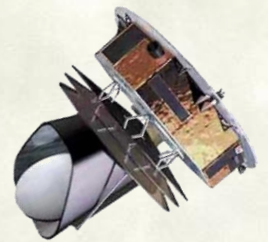
Planck : microwave
