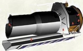
Spitzer : IR
